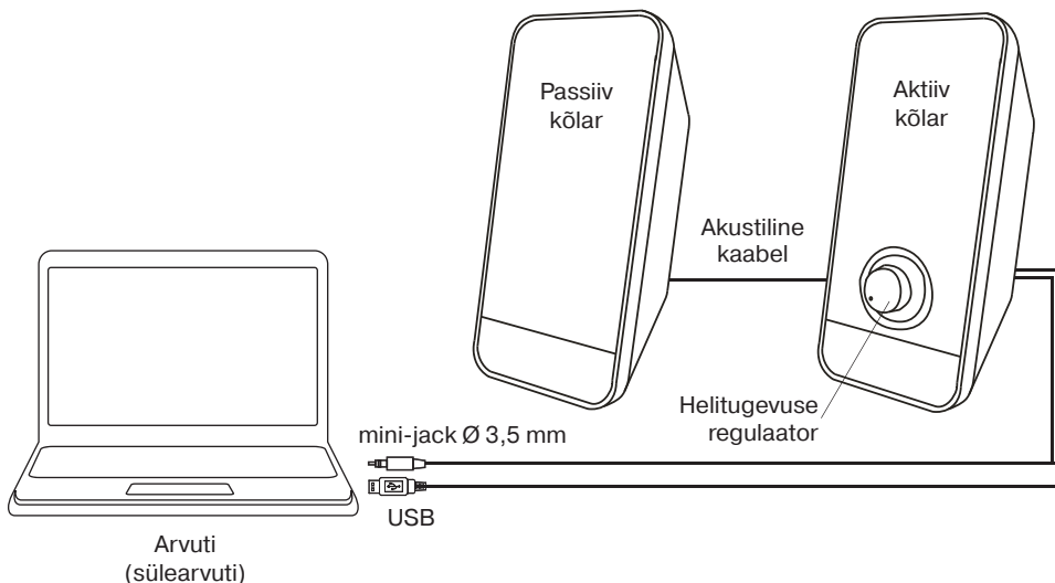
Joon. 2. Ühendamise skeem
